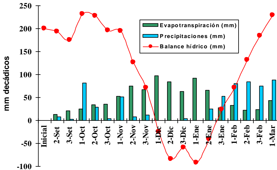
Figura 1: Precipitaciones, evapotranspiración y balance hídrico decádico acumulados (mm) en el sitio experimental. Wheelwright, Santa Fe. Agua disponible inicial en el suelo (200 cm) 200 mm. Precipitaciones totales en el ciclo 602,2 mm. Déficit acumulado de evapotranspiración 303 mm.
